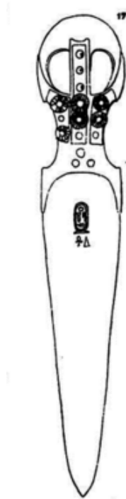
Dague en cuivre au cartouche de Souadjentrê Nebiryraou, dessin de Flinders Petrie, 1901.
